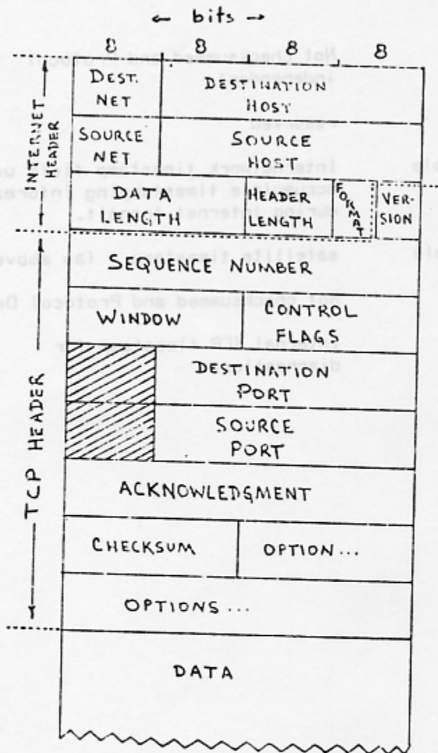
TCP Header Format
